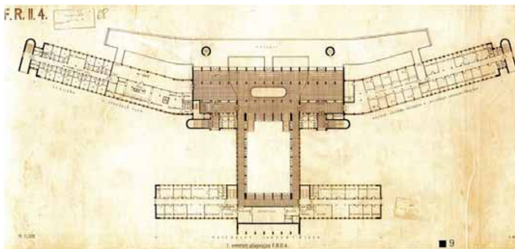
Ferihegy I. terminál alaprajza
