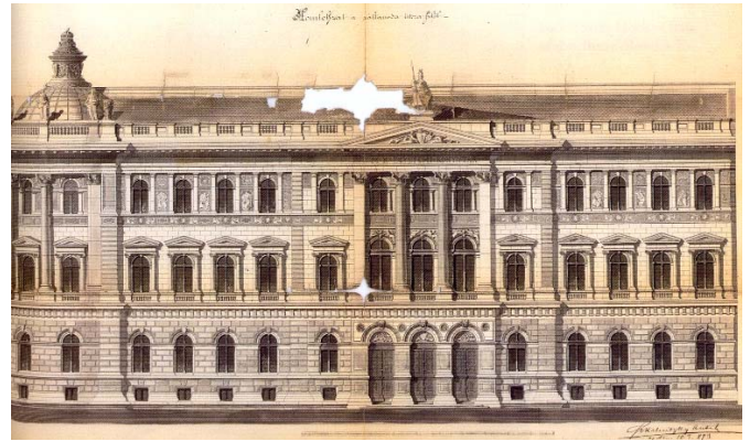
A magyar kir. tud. Egyetem könyvtárának homlokzati tervrajza (BFL)
